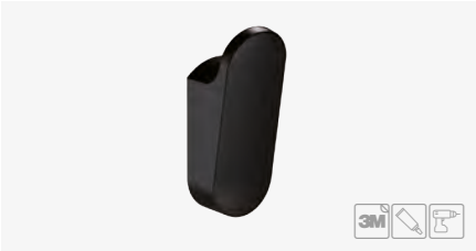
PERCHA S6 ● NEGRO ● CROMO A: 26 mm. B: 70 mm. C: 25 mm.
